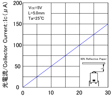
光電流-順電流特性
