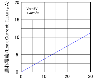
漏れ電流-順電流特性
