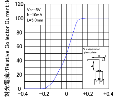
検出位置特性
