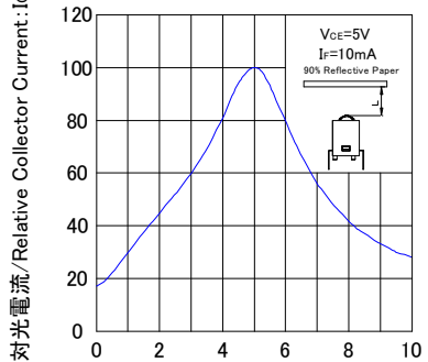
相対光電流-距離特性
